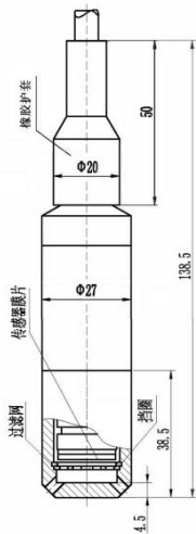
图 1 直接引线式
