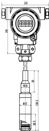
图 3 带显示 2088 壳体液位计
