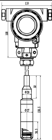
图 2 不带显示 2088 壳体液位计
